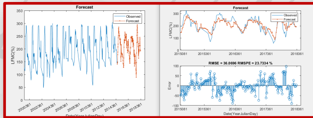
Figura 1 Modelo de predicción de LFMCI basado en LSTM, a partir de variables meteorológicas actuales y datos previos de LFMCI en California.
